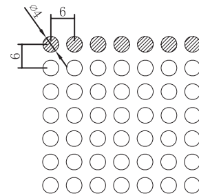
No. P26 | Max. width 726mm Thickness 0.4-0.7mm Open Area 34.9%
